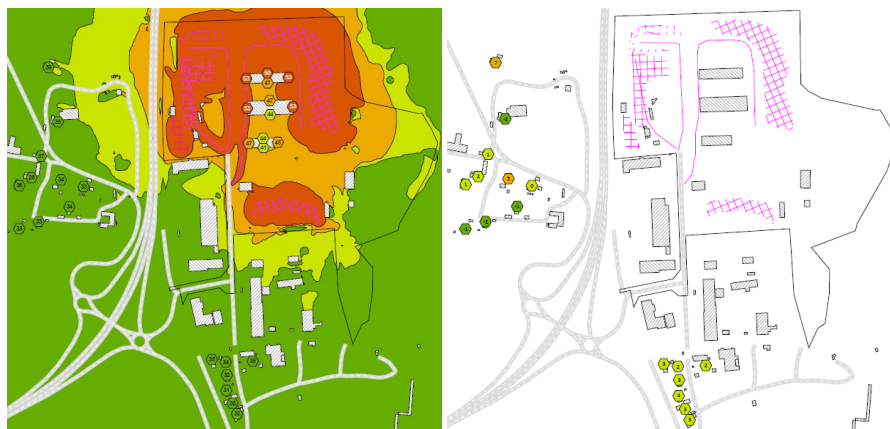
Figur 13. T.v.: Ekvivalent ljudnivå för verksamhetsbuller från planerad utbyggd ÅVC. T.h.: Skillnad i ekvivalent ljudnivå för verksamhetsbuller mellan utbyggnadsalternativet och nuläget.
