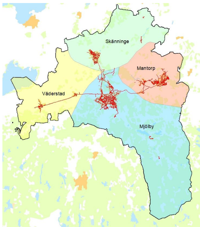
Figur 3 Översiktsbild ledningsnätets utbredning
