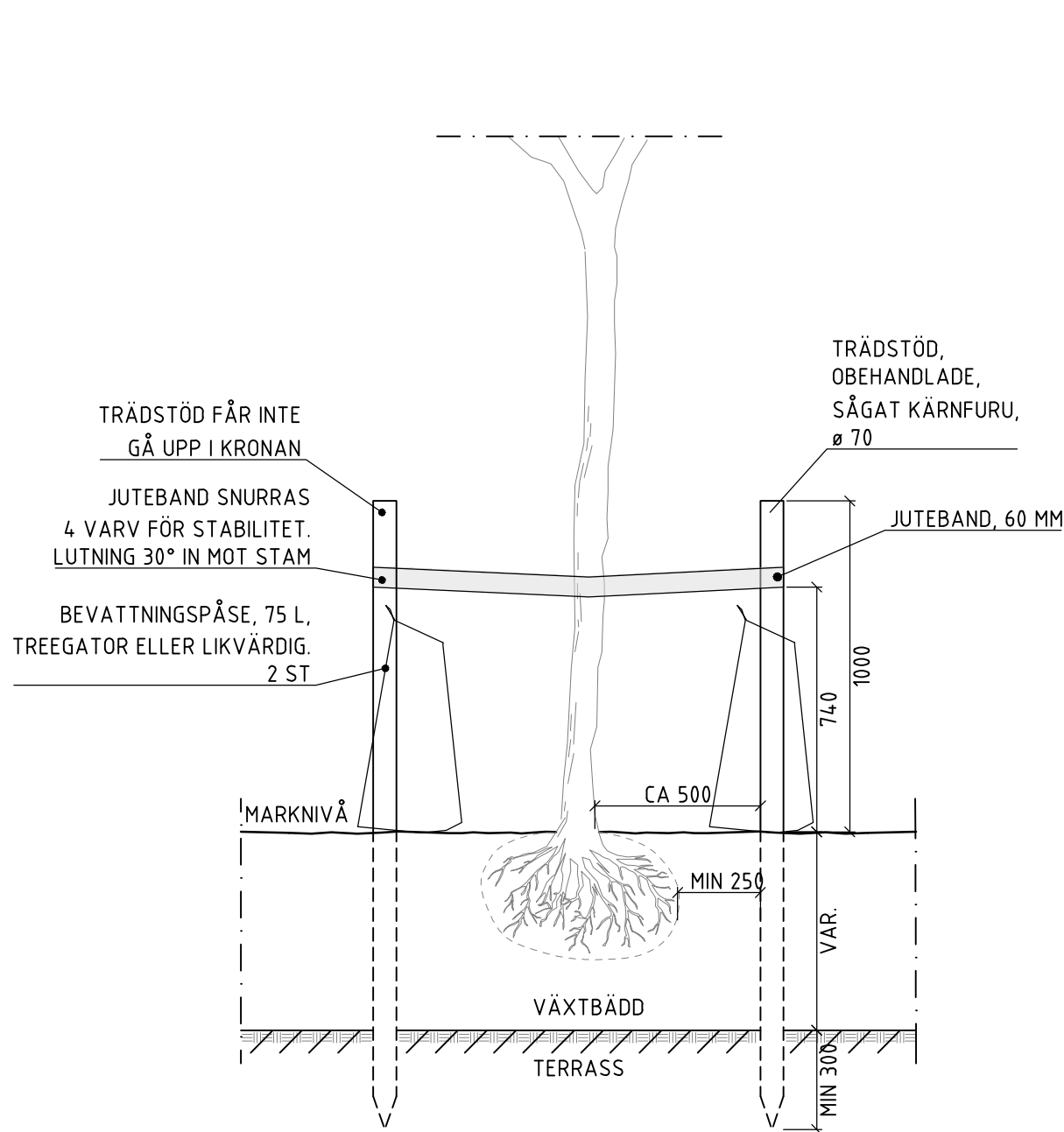
TS1 TRÄDSTÖD FÖR TRÄD I KVALITÉ UNDER 20 PRINCIPSEKTION SKALA 1:20
