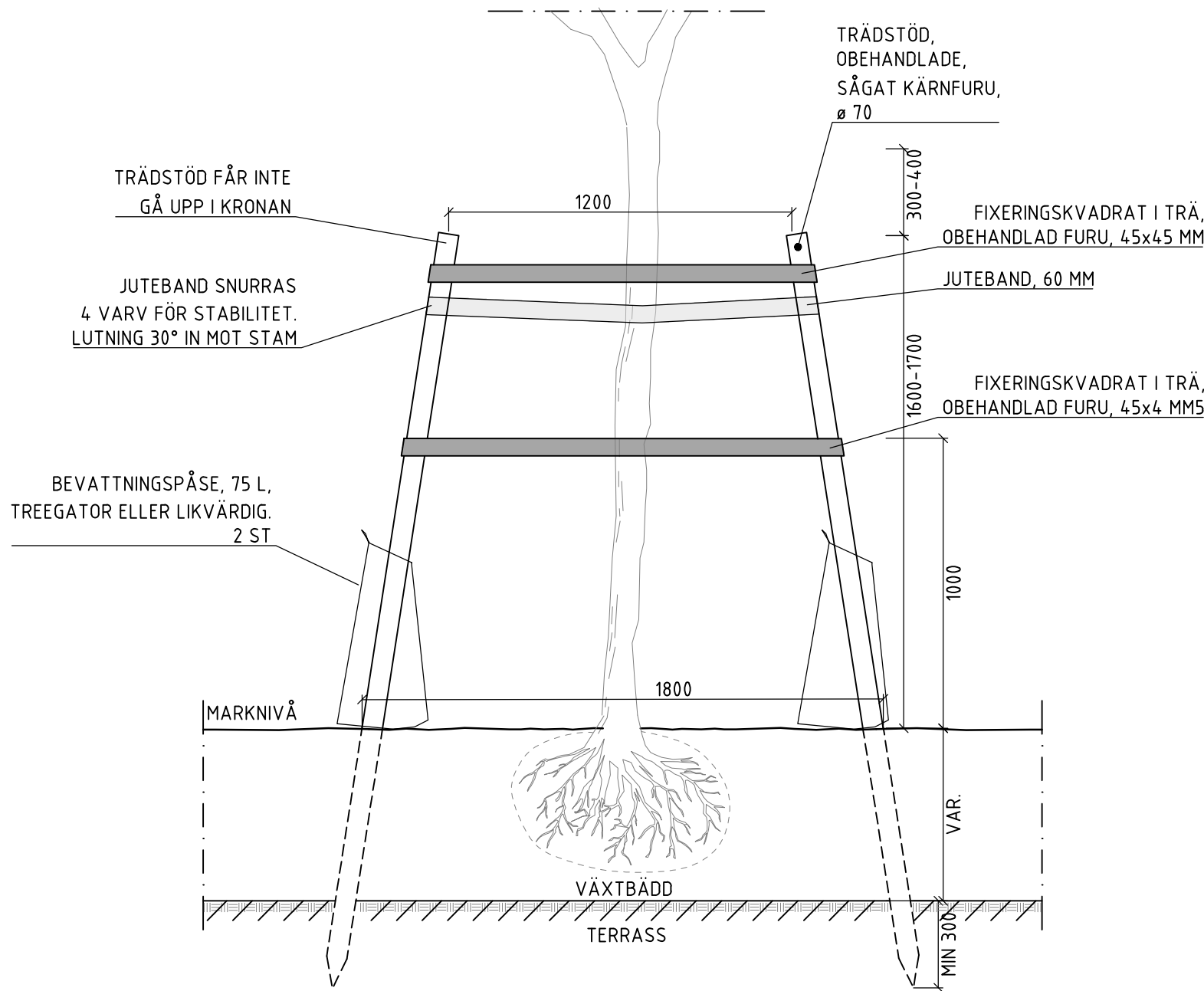
TS2 TRÄDSTÖD FÖR TRÄD I KVALITÉ 20-35 PRINCIPSEKTION SKALA 1:20
