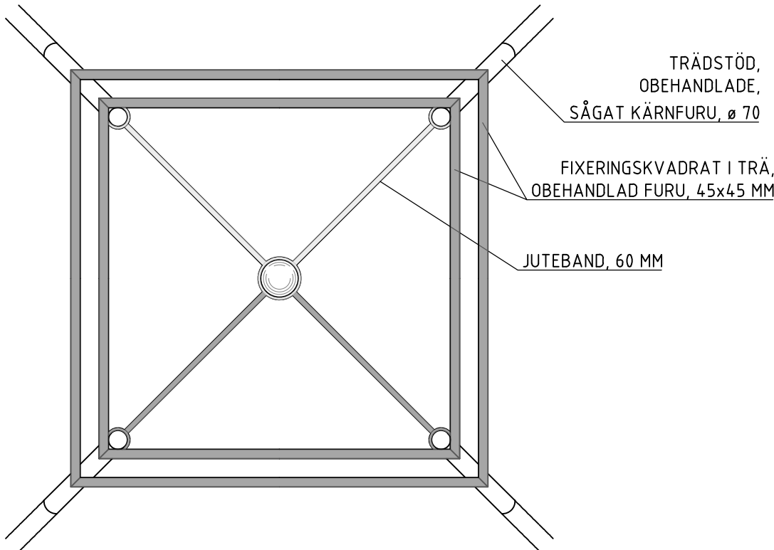
TS2 TRÄDSTÖD FÖR TRÄD I KVALITÉ 20-35 PLAN SKALA 1:20
