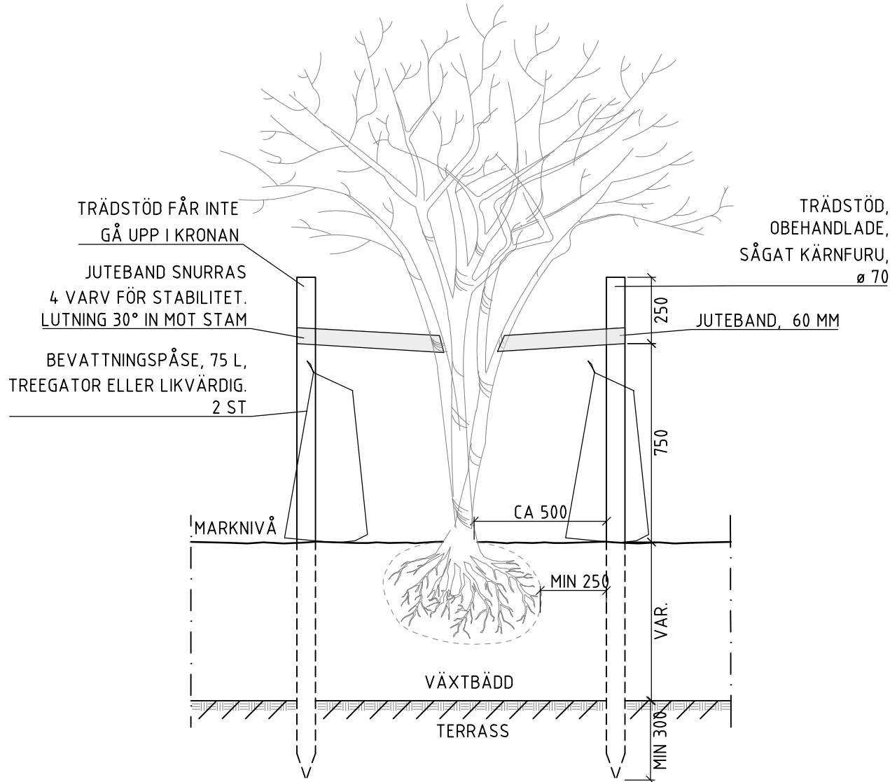
TS3 TRÄDSTÖD FÖR FLERSTAMMIGA TRÄD PRINCIPSEKTION SKALA 1:20
