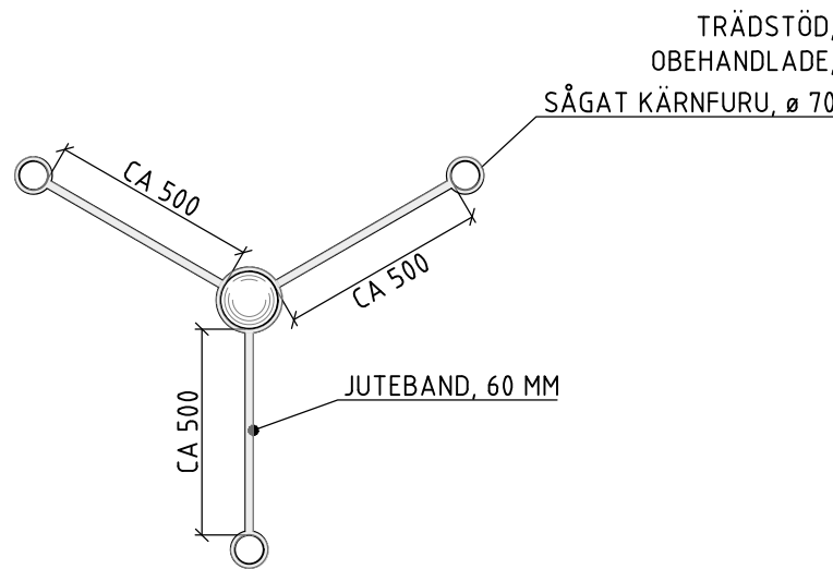
TS1 TRÄDSTÖD FÖR TRÄD I KVALITÉ UNDER 20 PLAN SKALA 1:20
