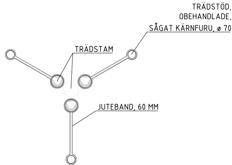
TS3 TRÄDSTÖD FÖR FLERSTAMMIGA TRÄD PLAN SKALA 1:20
