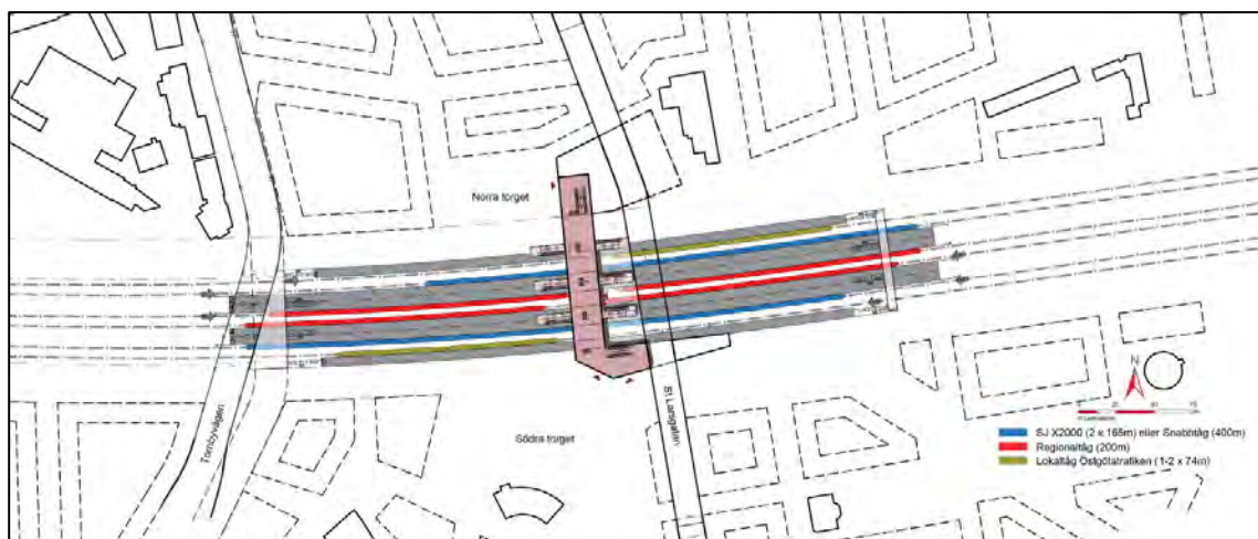
Figur 17 Princip för plattformar. Steningeviadukten och en förlängning av S:t Larsgatan föreslås kunna passera över spåren. Runt stationen kan Linköpings kommun planera för nya stads kvarter. Streckade linjer visar schematiskt hur kvarter skulle kunna tillkomma.
