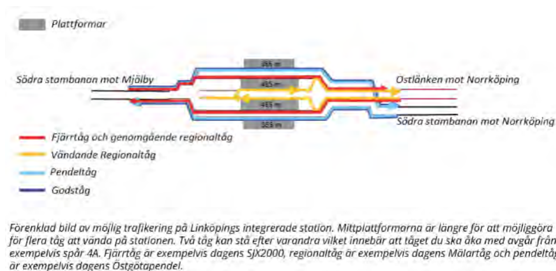
Figur 13 skiss över spår och plattformar för den nya stationen.
